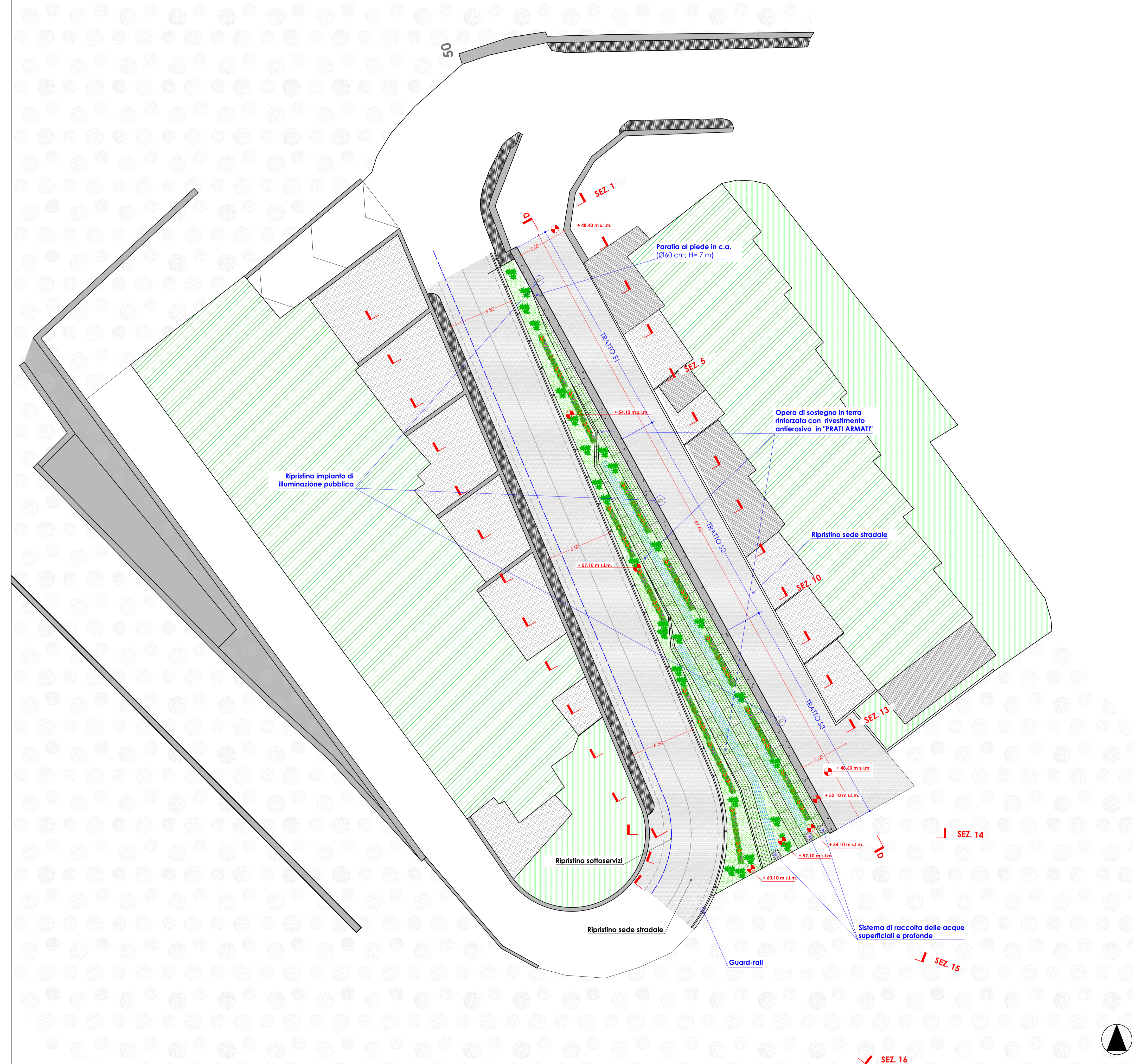
PLANIMETRIA STATO DI PROGETTO - SCALA 1: 200
