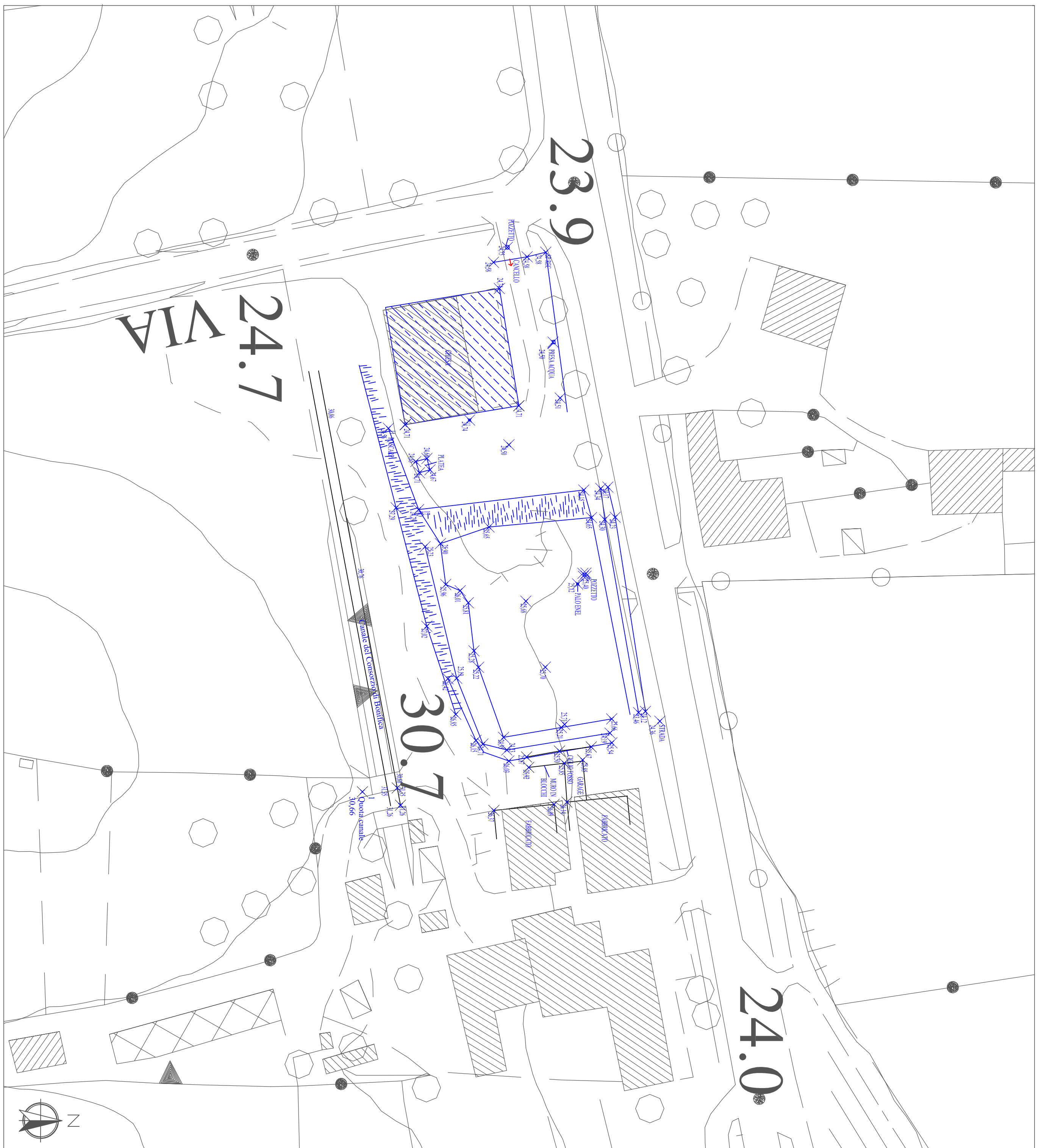
Piano quotato sovrapposto alla C.T.R. (Stato di fatto)
