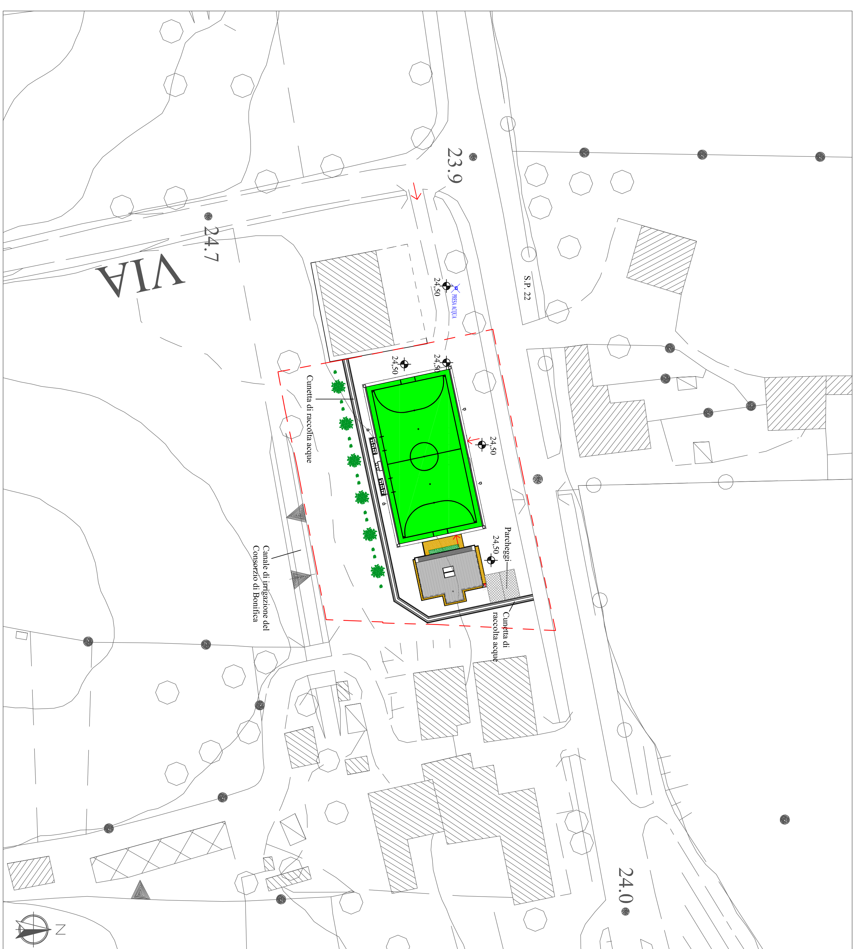
Planimetria generale (Stato futuro)
