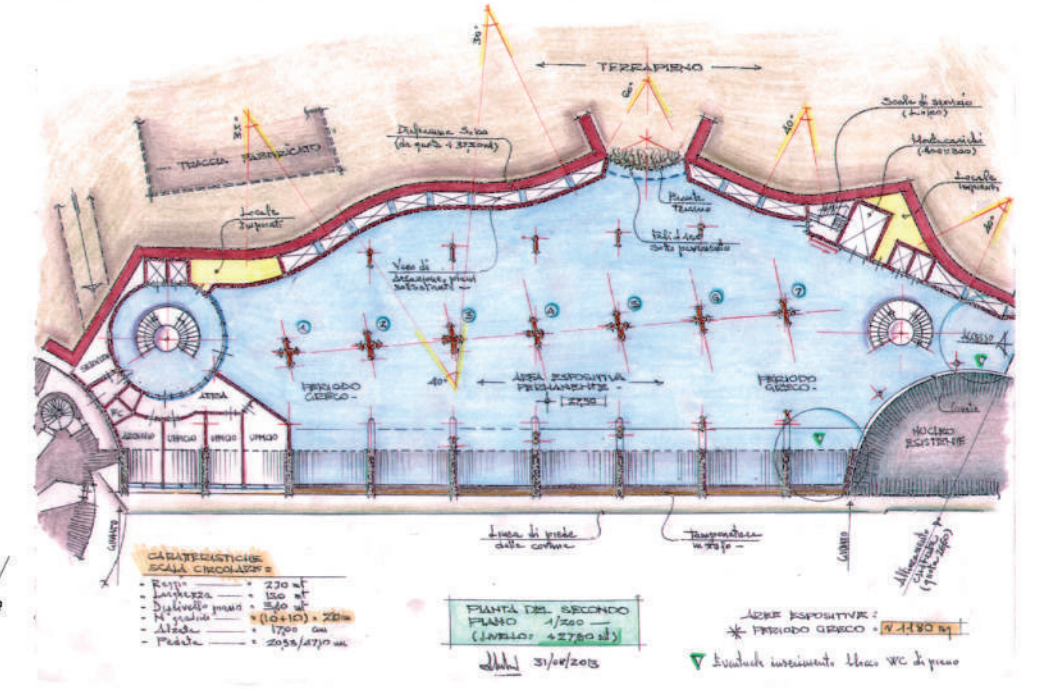
PIANTA DEL SECONDO ORIZZONTAMENTO (Quota estradosso: -2,77,75 mt) SCHEMA PLANIMETRICO CON LE PORZIONI D'IMPALCATO DA REALIZZARE IN FASE DI SCAVO. ALTI D'ETTERALI COSTRUTTIVI PIANTE GENERALI AL SECONDO PIANO (Dal brogliaccio di studio delle fasi preliminari) SCALA: 1/100-1/200
